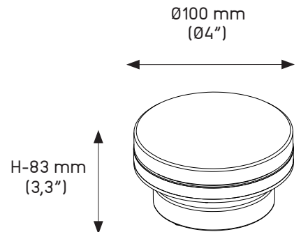
Trimless(TS)
